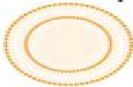
Liposome
