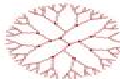
Dendrimer
