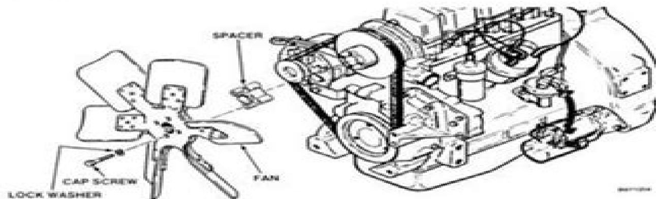
Fan Installation
