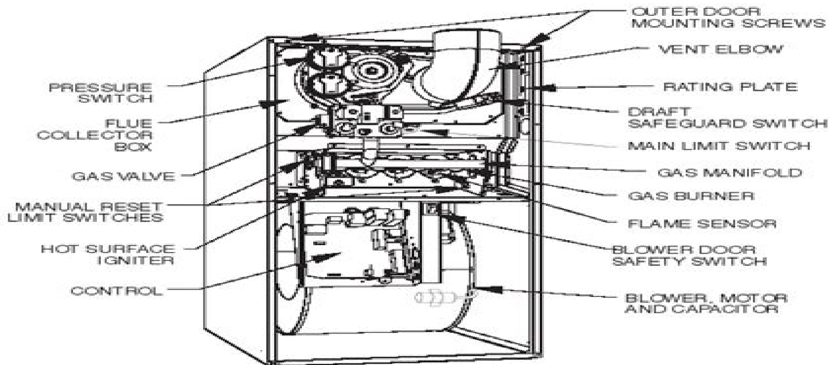
Fig. 3—Model 58 DT 5 Upflow
