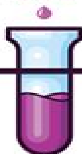
HEMERYTHRIN
