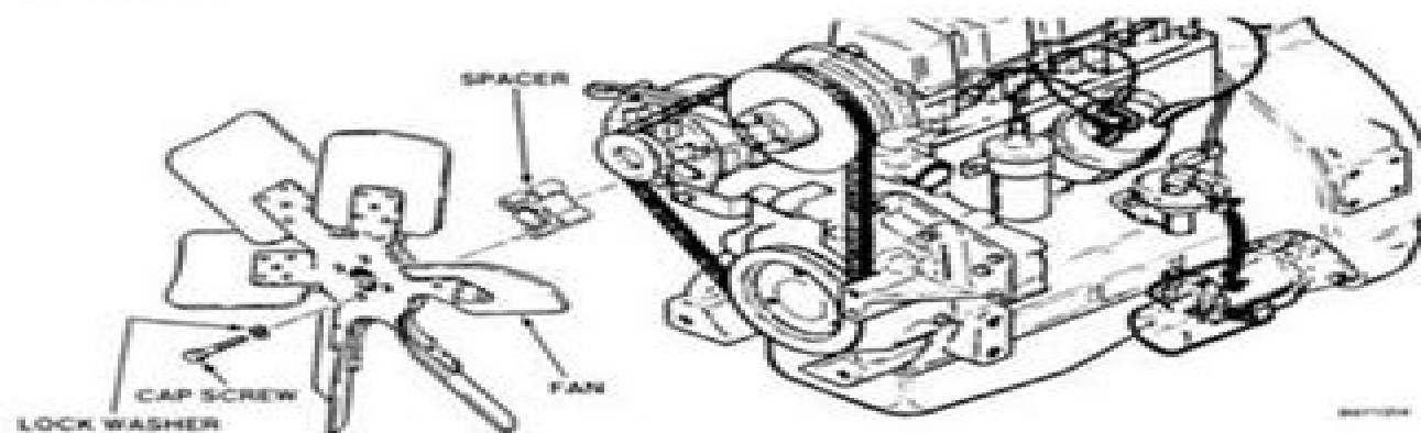
Fan Installation
